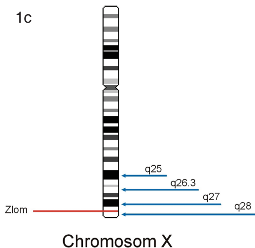
Obr. 1. Schematické znázornenie mapovania a určovania lokalizácie zlomu na chromozóme X u detskej pacientky s ALL asociovanou s prestavbou 11q23. Pomocou FISH sa potvrdila translokácia génu MLL s partnerským X chromozómom (nie je ukázané). A. Výsledok FISH s BAC sondou RP11-298A8, ktorá mapuje do oblasti Xq27 a je značená zeleným fluorochrómom, a zároveň s centromerickou sondou CEPX (Abbott-Vysis), ktorá je značená červeným fluorochrómom. Lokalizácia BAC sondy na X chromozóme potvrdzuje, že zlom nenastal v pruhu q27. B. Mapovanie oblasti Xq28 pomocou BAC sondy RP11-1085P10 značenej zeleným fluorochrómom a centromerickej sondy CEPX (Abbott-Vysis) značenej červeným fluorochrómom. Lokalizácia signálu BAC sondy na inom chromozóme (chromozóm 11) potvrdzuje zlom X chromozómu v pruhu q28. C. Mapa X chromozómu znázorňuje zlom v pruhu q28. Fúzia MLL génu s Xq28 nebola doteraz popísaná.
