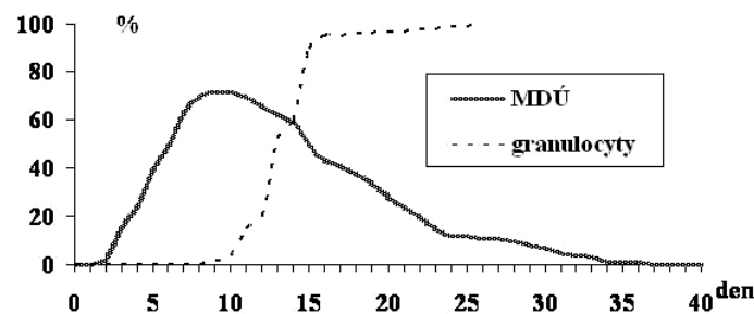
Graf 2. Incidence postižení mukozitidou dutiny ústní (MDÚ) v aktuální den po alogenní transplantaci krvetvorných buněk u protokolu přípravy FLU/MEL a incidence reparace granulopoézy (granulocyty \geq 1,0 \times 10^9/\text{l} ).
