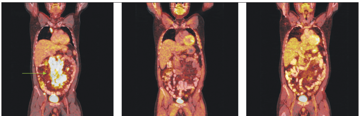
Obr. 1. Série PET/CT snímků u nemocného s difúzním B-velkobuněčným lymfomem před léčbou, po 2 cyklech léčby a po ukončení léčby. První snímek ukazuje mnohočetná ložiska hypermetabolismu glukózy ve zvětšených lymfatických uzlinách infraklavikulárně a v dutině břišní kolem břišní aorty a v mezenteriu a kolem pánevních cév. Po 2 cyklech léčby došlo ke zmenšení všech lymfatických uzlin, žádná nevykazuje hypermetabolismus glukózy a po skončení léčby je patrná normalizace velikosti lymfatických uzlin, všechny bez hypermetabolismu glukózy.
