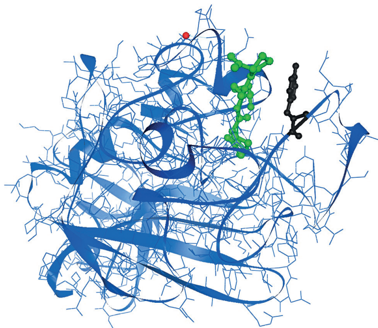
Obr. 4. Krytalografická struktura γC domény s GPRP peptidem navázaným v polymeračním místě „a“ γ Tyr363 (černě) je součástí polymerační prohlubně „a“ γC domény. GPRP peptid je znázorněn zeleně. Červeně je zvýrazněn ion Ca 2+ .
