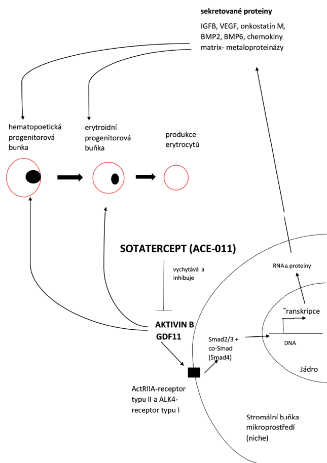
Obr. 3. Mechanismus působení sotaterceptu (ACE-011) na hematopoetickou progenitorovou buňku a erytroidní progenitorovou buňku diferencující na erytrocyty inhibicí signální dráhy GDF 11 a aktivinu B ve stromální buňce mikroprostředí (niche)
