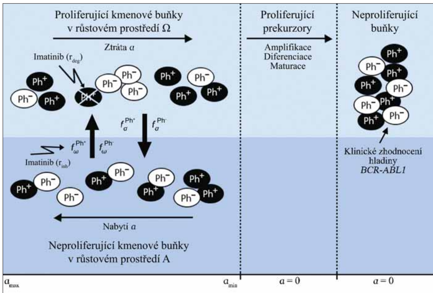
Obr. 1. Schéma ABM modelu. Předpokládá se koexistence zdravých ( Ph^- ) a maligních ( Ph^+ ) kmenových buněk ve dvou prostředích růstu ( A , \Omega ). Náclonost buněk k výskytu v prostředí A je dána jejich afinitou ( \alpha ). V prostředí \Omega dochází k postupné ztrátě \alpha , v prostředí A naopak k jejímu znovunabytí. Buňky, které ztratily svůj potenciál pobývat v prostředí A (jejich \alpha < \alpha_{min} ) jsou označeny jako diferencované. Ty vytvářejí klon, který přechodně expanduje (proliferující prekurzory). Tento klon, který existuje po fixně stanovenou dobu bez další expanze, představuje neproliferující prekurzory a terminálně diferencované buňky (neproliferující buňky). Aktivní proliferace kmenových buněk je možná pouze v prostředí \Omega . Přechod Ph^- a Ph^+ buněk mezi těmito prostředími je dán charakteristikou f_{\alpha}^{Ph^-} , f_{\alpha}^{Ph^+} , f_{\omega}^{Ph^-} , f_{\omega}^{Ph^+} . Předpokládá se dvojitý specifický efekt imatinibu na Ph^+ buňky: inhibice proliferace r_{inh} (efekt na f_{\omega}^{Ph^+} ) a degradace proliferujících kmenových buněk r_{deg} . Upraveno dle [21].
