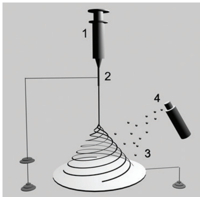
Obr. 1 Elektrostatičké zvlákňování bylo prováděno v laminárním boxu kvůli zajištění sterilních podmínek. Polymerní roztok byl umístěn ve stříkačce (1) s kladně nabitou jehlou (2). Vznikající nanovláknina byla sbírána na uzemněný kolektor (3). Suspenze trombocytů (4) byla sprejována mezi vznikající nanovláknina v 5minutových intervalech během celého procesu zvlákňování.
