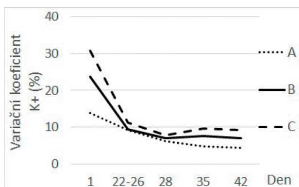
Graf 6 Závislost hladiny variačního koeficientu kalia na době skladování v podskupinách
