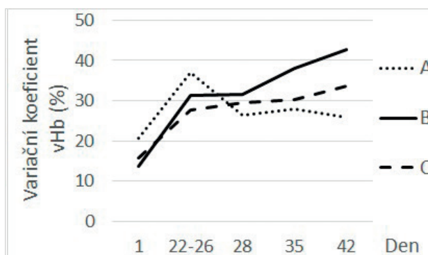
Graf 5 Závislost hladiny variačního koeficientu volného hemoglobinu na době skladování v podskupinách
