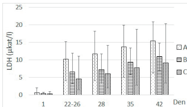
Graf 3 Závislost hladiny LDH na době skladování v podskupinách. Spočítáno jako aritmetický průměr s rozmezím minimální a maximální změřené hodnoty.
