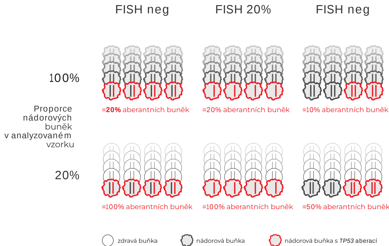
Obr. 1. Podíl nádorových buněk nesoucích TP53 abraci při výsledku sekvenování nové generace \approx 10\% VAF v závislosti na proporci nádorových buněk ve vzorku a stavu druhé alely. (A) Poškození jedné alely mutací. Druhá alela může být intaktní nebo vyražena nezávislou mutací. (B) Kombinace mutace jedné alely a delecí druhé alely detekované pomocí FISH (VAF = 11,1 %). (C) Obě alely mutované mechanismem zdvojení mutované alely cnLOH.
